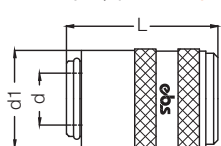
Адаптер муфты / Adapter Socket
