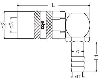
Муфта 90° под шланг / 90° Hose Tail Socket
