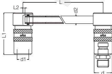
Соединитель с муфтами / Diverting Socket
