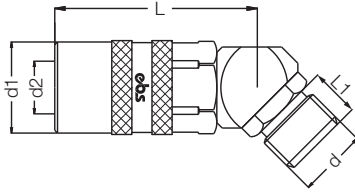
Муфта 45° с наружной резьбой / 45° Male Thread Socket
