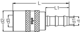
Муфта прямая под шланг с бесхомотовым соединением / Flex Hose Tail Socket
