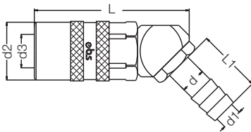
Муфта 45° под шланг / 45° Hose Tail Socket
