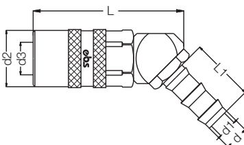
Муфта 45° под шланг с бесхомотовым соединением / 45° Hose Clamp Socket
