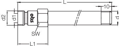
Удлинительный ниппель с резьбой / Extension Plug With Thread
