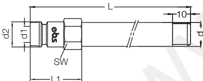
Удлинительный ниппель с резьбой / Extension Plug With Thread
